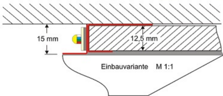
Einbauvariante TYP-C_FLEX
