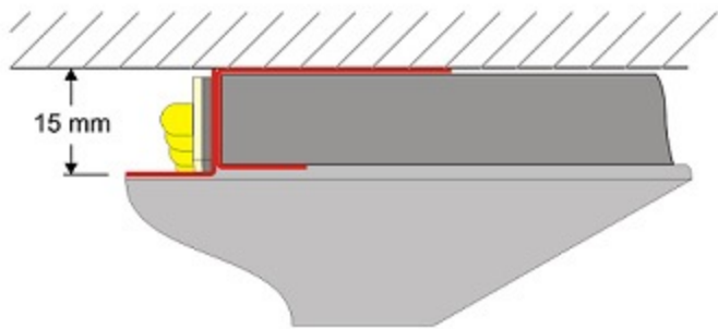
Einbauvariante TYP-C_FLEX
